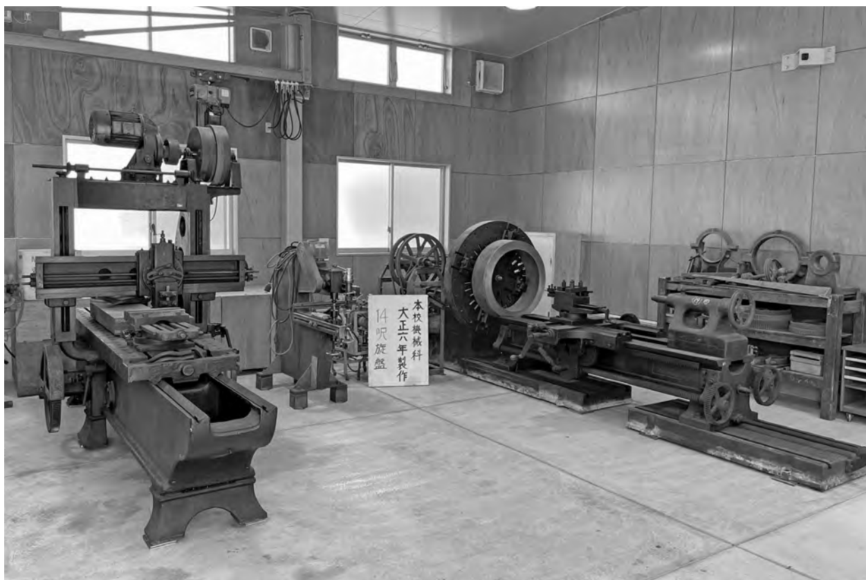
大正6年に本校機械科が製作した14呎旋盤
